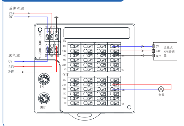
EC5-I08C-008P-A (NPN输入,PNP输出)
