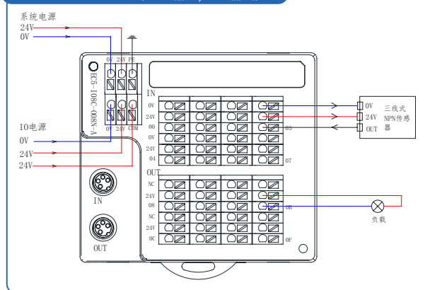
EC5-I08C-008N-A (NPN输入,NPN输出)
