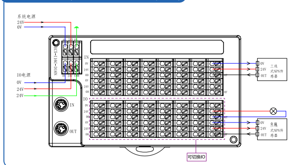
EC5-I16C-D16N(NPN输入, NPN输入/输出)
