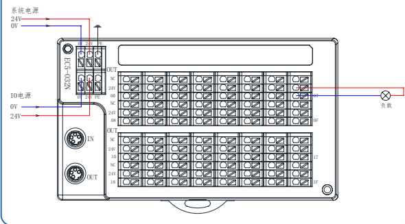
EC5-O32N (NPN输出)
