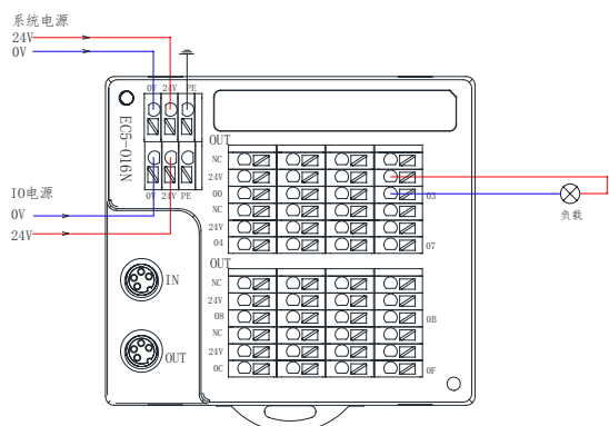
EC5-O16N (NPN输出)
