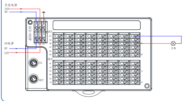
EC5-O32P (PNP输出)
