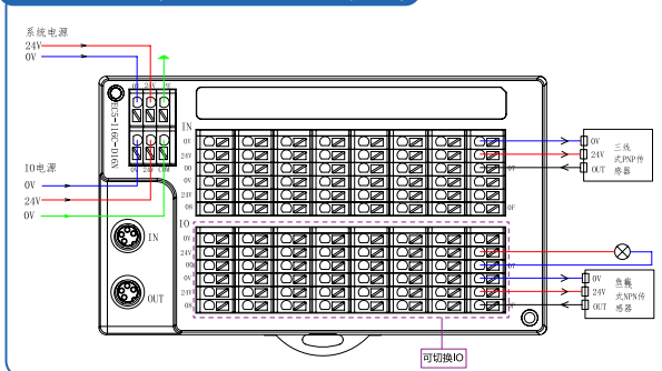
EC5-I16C-D16N(PNP输入, NPN输入/输出)
