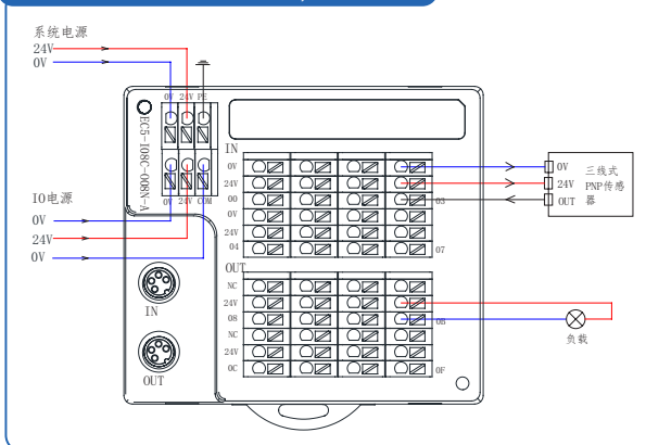
EC5-I08C-008N-A (PNP输入,NPN输出)
